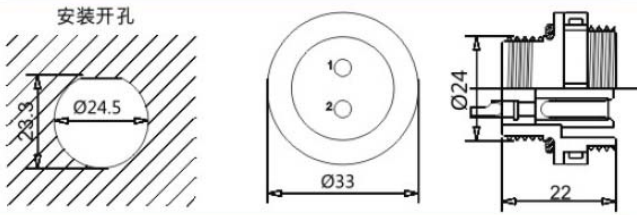
2 孔法兰插座: ZS
