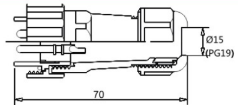
直式软管插头: TR
