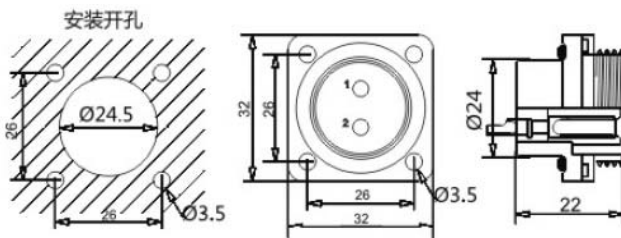
电缆对接插座: ZP
