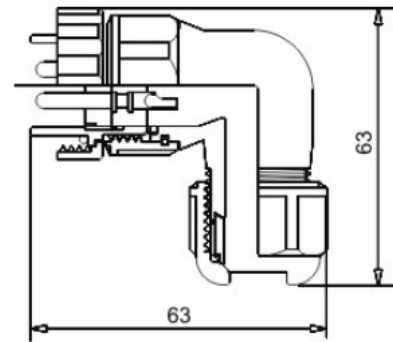
弯式软管插头: TC
