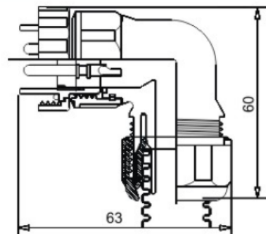
直式电缆插头: TP
