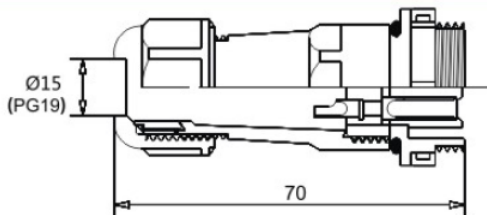
直式软管插座: ZR
