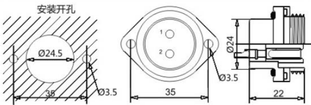
方盘法兰插座: ZG
